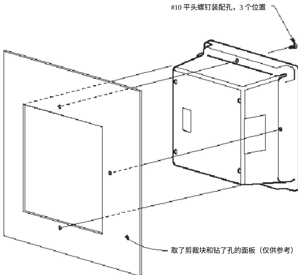
图 33 面板安装
